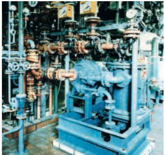
Gaspumpen-Kompaktanlage Typ FGP aus Keramik / PTFE / Hastelloy zur Verdichtung korrosiver Gase vor der Verbrennungsanlage
